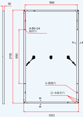
背面図
